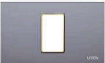
VPROMAX-PM1 152.000 VND Mặt dùng cho 1 thiết bị cỡ S Vpromax UTEN Kích thước: 117x74mm Chất liệu: Gông sắt sơn tĩnh điện, Mặt kính Đóng gói: Cái/ hộp
